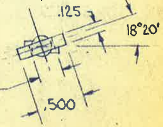
# CROSS-BAR LOWER LINK STEEL 1 L.H. & 1 R.H. REQD ✓
