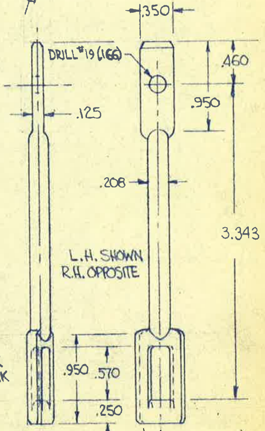
# CROSS-BAR LOWER LINK STEEL 1 L.H. & 1 R.H. REQD ✓
