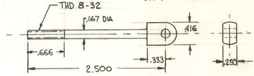
#9145 T.T. HANGER STEEL 2 REQD
