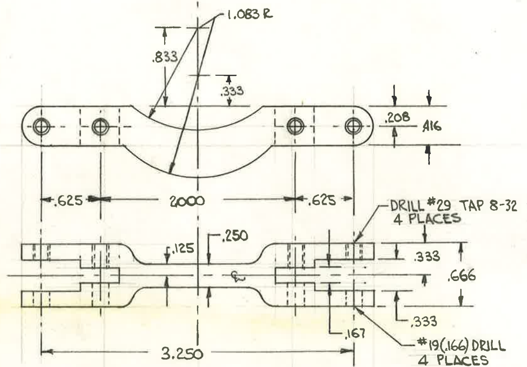
#7145 TRANSVERSE EQUALIZER STL 1 REQD
