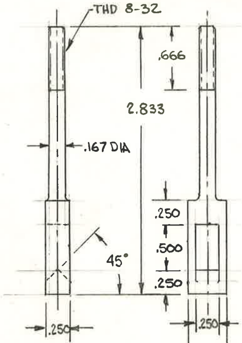
#9145 T.T. HANGER STL 2 REQD
