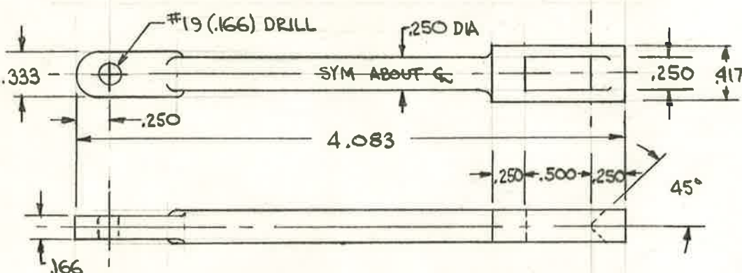
#8145 T.T. HANGER STEEL 2 REQD
